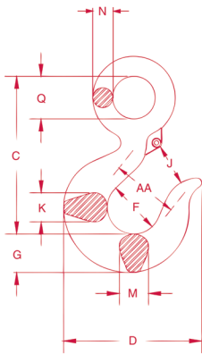
L-320N EYE HOOK
